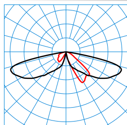
LTX K-AB2L-LR/1800-730 2G1 ET TX776427
