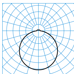
Olisq RWD4 DW 40-8TW ETDD8 IP54 (DSU) TX874154
