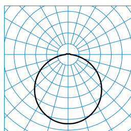
Olisq RWD4 DW 40-8TW ETDD8 IP54 + Olisq RWD4 C 01 (DWW) TX874158
