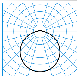
Olisq RWD4 DW 40-8TW ETDD8 IP54 (DWW) TX874155
