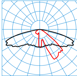
Publisca P1W-AB2L/1800-740 2G1S TX053464
