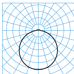
Olisq RWD2 DW 14-40/4/ML-830 IP54 ET + Olisq RWD2 ZDR 1/2 01 (stage 0) TX778195
