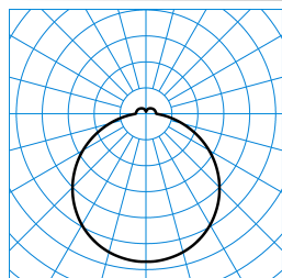
Olisq RWD2 DW 14-40/4/ML-830 IP54 ET (stage 0) TX778113
