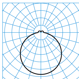
Olisq RWD2 DW 14-40/4/ML-830 IP54 ET (stage 1) TX778116
