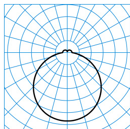
Olisq RWD2 DW 14-40/4/ML-830 IP54 ET (stage 2) TX778121
