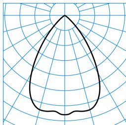
InperlaL G2 C07 BR25 4700-840 ETDD 03 ■ C0 - C180 TX769261
