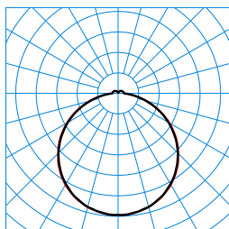
Olisq QWD3 DW 30-840 ETBLE +DMM IK + Olisq QWD3 ZDR 1/2 05 TX461644
