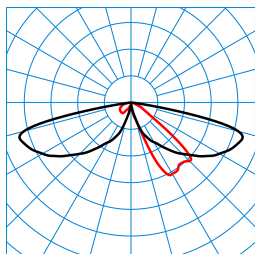
LTX L-AB2L-LRA/15/18/26-730 4G1 (1500 lm) TX076486
