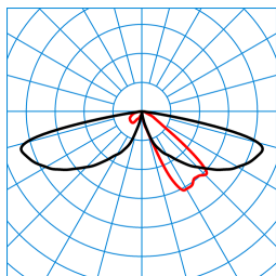
LTX L-AB2L-LRA/15/18/26-730 4G1 (2600 lm) TX779564
