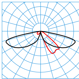
LTX L-AB2L-LRA/15/18/26-730 4G1 (1800 lm) TX779560
