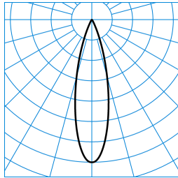
7651 LentyP L-MF 20-827 M32 ET 05 (150) TX782240
