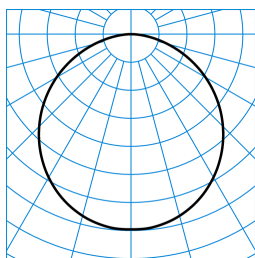
Olisq RWD2 DW 20-840 ET EB3 IP54 PC + Olisq RWD2 ZDR 1/1 01 TX425914
