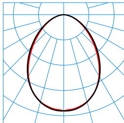
SFlow D3-L MRWD LED4000-840 ETDD LLWM 01 TX770236
