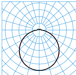
Olisq QWD2 DW 35-840 ET HFS + Olisq QWD2 ZDR 1/2 01 TX462397
