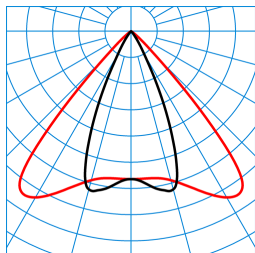
E-Line 7651 Grado WRS-DF84 50-835 M42 ETDD 03 (225) TX845269
