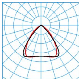
ELINE LN55-140 ML 840 L225 0 50
