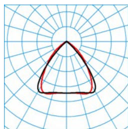
ELINE LN55-140 ML 840 L225 2 50
