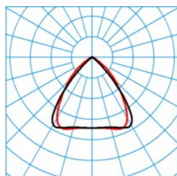
ELINE LN55-140 ML 840 L225 4 50
