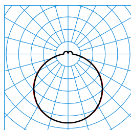
Olisq QWD2 DW 35-8TW ETDD8 IK (DSU) TX873206
