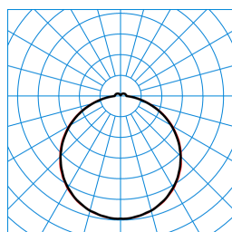
Olisq QWD2 DW 35-8TW ETDD8 IK + QWD2 ZDR 1/2 01 (DWW) TX873219
