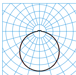
Olisq QWD2 DW 35-8TW ETDD8 IK + QWD2 ZDR 1/2 03 (DWW) TX873222
