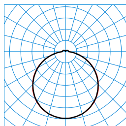
Olisq QWD2 DW 35-8TW ETDD8 IK + QWD2 ZDR 1/2 05 (DWW) TX873225
