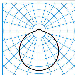
Olisq QWD2 DW 35-8TW ETDD8 IK (DWW) TX873207
