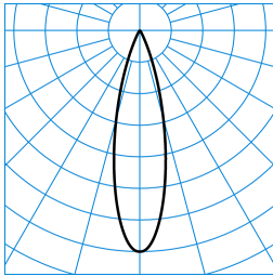
7651 LentyP L-MF 40-EC M39 ETDD 05 (150) TX782168
