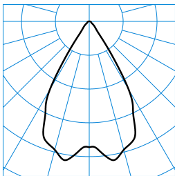
InperlaLP C05 HR19 1800-940 01 + ZN-PC ■ C0 - C180 TX045486
