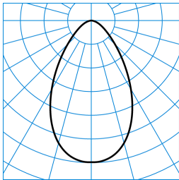
InperlaLP C05 HR19 1800-940 01 + DA-M 03 ■ C0 - C180 TX045483
