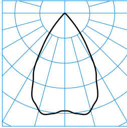
InperlaLP C05 HR19 1800-940 ETDD 01 ■ C0 - C180 TX768237
