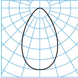
InperlaLP C05 HR19 1800-940 01 + DA-M 01 ■ C0 - C180 TX045482
