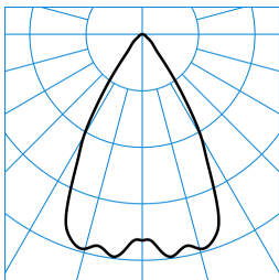
InperlaLP C05 HR19 1800-940 01 + RG-PC ■ C0 - C180 TX045485
