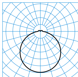
Olisq RWD3 DW 30-840 ETBLE +DMM IP54 PC + Olisq RWD3 ZDR 1/2 05 TX426269
