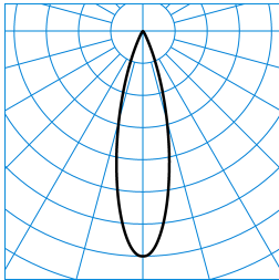
7651 LentyP L-MF 30-BC M49 ETDD 01 (225) TX782009
