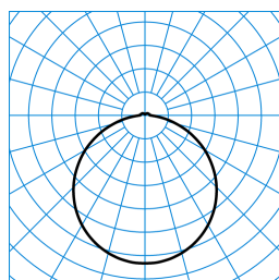
Olisq RWD4 DW 40-830 ETBLE +DMM IP54 + Olisq RWD4 ZDR 1/2 01 TX427264
