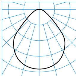
Onplana D11 CDP19 4000-8TW ETDD8 01 (DCW) TX874439
