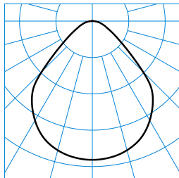
Onplana D11 CDP19 4000-8TW ETDD8 01 (DWW) TX874441
