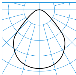
Onplana D11 CDP19 4000-8TW ETDD8 01 (DSU) TX874440
