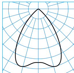
InperlaL G2 C07 BR19 1800-840 03 + DA 03 ■ C0 - C180 TX052828
