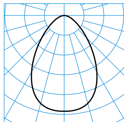
InperlaL G2 C07 BR19 1800-840 03 + DA-M 03 ■ C0 - C180 TX052829
