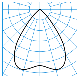
InperlaL G2 C07 BR19 1800-840 ETDD 03 ■ C0 - C180 TX768218
