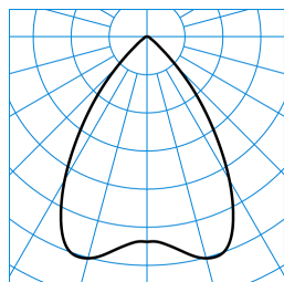
InperlaL G2 C07 BR19 1800-840 03 + RD-PC ■ C0 - C180 TX052830
