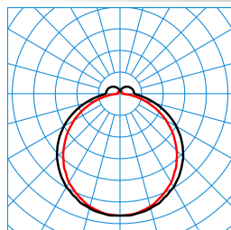
Olisq LWD2 DW 40-840 ETDD IP54 PC TX376325
