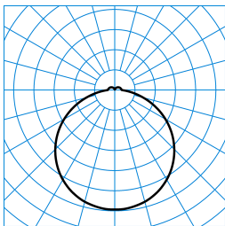
Olisq RWD3 DW 30-840 ET HFS IP54 PC + Olisq RWD3 ZDR 1/2 05 TX42622
