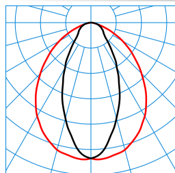
Nextrema G3 TB 8000-840 ET +LV PC TX770429
