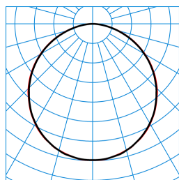
Olisq QWD2 DW 35-840 ETBLE +DMM + Olisq QWD2 ZDR 1/1 03 TX461484
