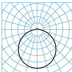
Olisq QWD2 DW 35-840 ETBLE +DMM + Olisq QWD2 ZDR 1/2 05 TX461592
