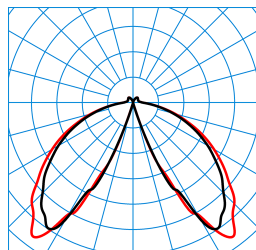
8841 RB/850-740 G2 ETDD (CLOANFANGSWERT) TX369204
