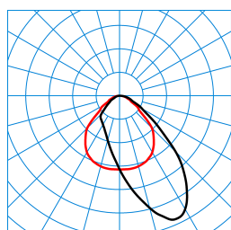
Luceos D/H2-L CDP-A 5000-830 ETDD 03 (Ceiling D2 ZD/03+EB3) TX877155
