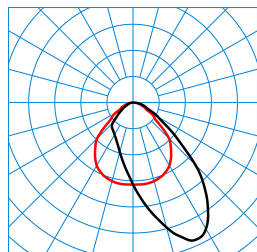
Luceos D/H2-L CDP-A 5000-830 ETDD 03 (Ceiling D2 ZD/03) TX877267
