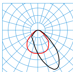
Luceos D/H2-L CDP-A 5000-830 ETDD 03 (Pendant ZS/ZST+EB3) TX877153
