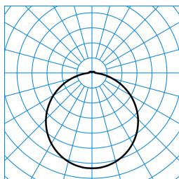
Olisq RWD4 DW 40-840 ETBLE +DMM + Olisq RWD4 ZDR 1/2 01 TX427287
