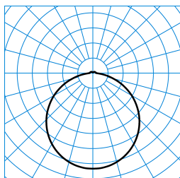
Olisq RWD4 DW 40-830 ET + Olisq RWD4 ZDR 1/2 03 TX427416
