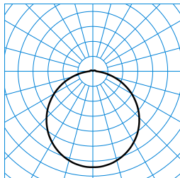
Olisq RWD4 DW 40-830 ET + Olisq RWD4 C 01 TX427011
