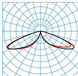
LTX KT-RB6L-LR/2600-730 3G1 ET TX780822
