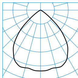
InperiaL G2 C07 BR22 1800-840 03 + RD-PC TX052890
