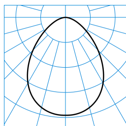
InperiaL G2 C07 BR22 1800-840 03 + DA-M 03 TX052889
