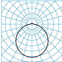
Olisq RWD4 DW 40-8TW ETBLE +CAS IP54 (DWW) TX876887
