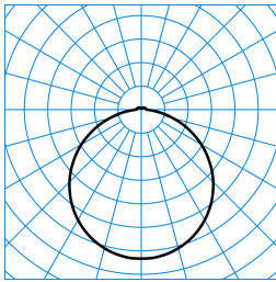
Olisq RWD4 DW 40-8TW ETBLE +CAS IP54 + Olisq RWD4 ZDR 1/2 03 (DWW) TX876803
