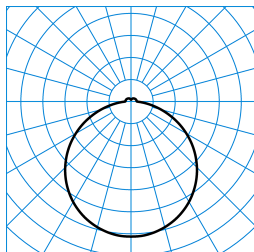
Olisq RWD4 DW 40-8TW ETBLE +CAS IP54 (DSU) TX876843
