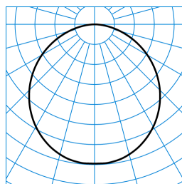
Olisq RWD1 DW 20-840 ET IP54 PC + Olisq RWD1 ZDR 1/1 01 TX425653
