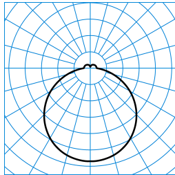
Olisq RWD2 DW 14-40/4/ML-840 ET PC (stage 2) TX842847
