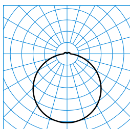
Olisq RWD2 DW 14-40/4/ML-840 ET PC + Olisq RWD2 ZDR 1/2 01 (stage 0) TX842959
