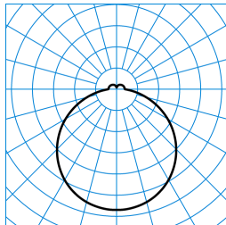
Olisq RWD2 DW 14-40/4/ML-840 ET PC (stage 3) TX842849
