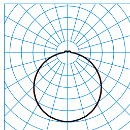
Olisq QWD3 DW 45-8TW ETDD8 + QWD3 ZDR 1/2 01 (DWW) TX873372
