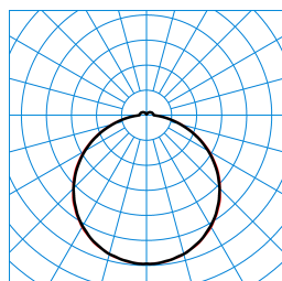
Olisq QWD3 DW 45-8TW ETDD8 + QWD3 ZDR 1/2 03 (DWW) TX873375
