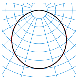
Olisq QWD2 DW 20-830 ET HFS IP54 IK + Olisq QWD2 ZDR 1/1 03 TX461423
