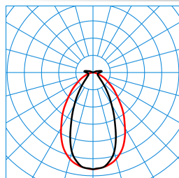
AragF 15 PN 64-840 ET PC LT TX769253
