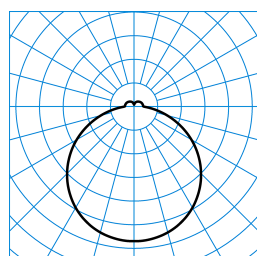
Olisq RWD2 DW 40-8TW ETDD8 (DSU) TX873641
