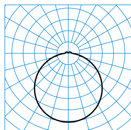
Olisq RWD2 DW 40-8TW ETDD8 + RWD2 ZDR 1/2 03 (DWW) TX873660
