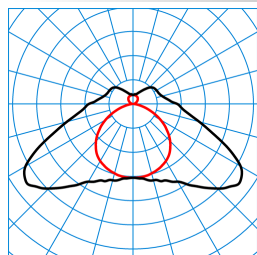
Tugra 12 PXW 45-840 ETDD PC C2 TX781520
