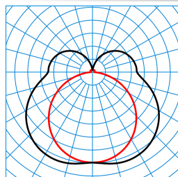
Montigo 600 O 1500-830 ET TX773625
