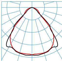
SFlow D2-L MRW LED4000-8TW ETDD8 01 (DSU) TX877016
