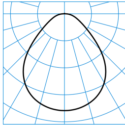
Onplana D07 CDP19 1000-830 ETDD 01 TX771512
