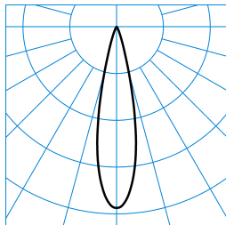
7651 Lentyp L-SP 40-830 M33 ETBLE 01 (225) TX782493
