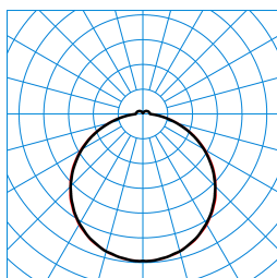
Olisq QWD3 DW 45-8TW ETDD8 IP54 IK + QWD3 ZDR 1/2 03 (DWW) TX873438
