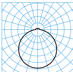
Olisq QWD3 DW 45-8TW ETDD8 IP54 IK (DSU) TX873422
