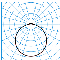
Olisq QWD3 DW 45-8TW ETDD8 IP54 IK (DWW) TX873423
