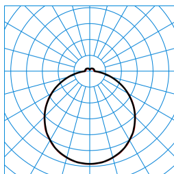
Olisq QWD3 DW 45-8TW ETDD8 IP54 IK (DCW) TX873421
