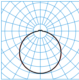
Olisq QWD3 DW 45-8TW ETDD8 IP54 IK + QWD3 ZDR 1/2 05 (DWW) TX873441
