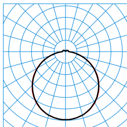
Olisq QWD3 DW 45-8TW ETDD8 IP54 IK + QWD3 ZDR 1/2 01 (DWW) TX873435
