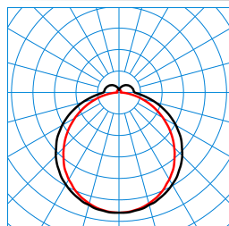
Olisq LWD3 DW 30-75/4/ML-830 ET IP54 (stage 0) TX460658
