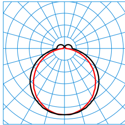
Olisq LWD2 DW 40-830 ETBLE +DMR IP54 TX376028
