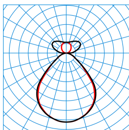
Opendo H2-L PW19 20-64/6/ML-830 ET 03 (2700lm) TX376589
