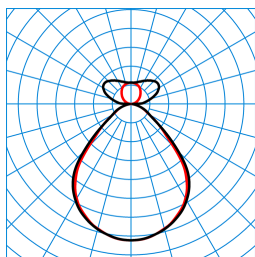
Opendo H2-L PW19 20-64/6/ML-830 ET 03 (4100lm) TX376590
