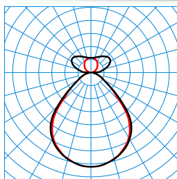
Opendo H2-L PW19 20-64/6/ML-830 ET 03 (2000lm) TX376584
