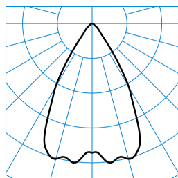
InperlaLP C05 HR19 1000-840 03 + RD-PC ■ C0 - C180 TX041637
