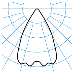
InperlaLP C05 HR19 1000-840 03 + RG-PC ■ C0 - C180 TX041638
