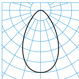
InperlaLP C05 HR19 1000-840 03 + DA-M 03 ■ C0 - C180 TX041636
