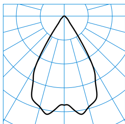
InperlaLP C05 HR19 1000-840 03 + ZN-PC ■ C0 - C180 TX041639
