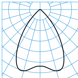
InperlaL G2 C07 BR19 2700-840 03 + RD-PC ■ C0 - C180 TX052854
