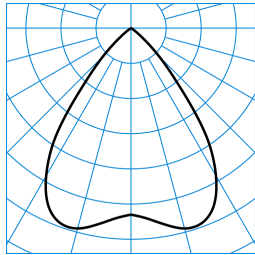
InperlaL G2 C07 BR19 2700-840 ETDD 03 ■ C0 - C180 TX768373
