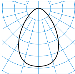
InperlaL G2 C07 BR19 2700-840 03 + DA-M 03 ■ C0 - C180 TX052853
