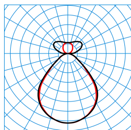
Opendo H2-L PW19 20-64/6/ML-840 ET 03 (2800lm) TX376532
