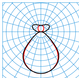
Opendo H2-L PW19 20-64/6/ML-840 ET 03 (4300lm) TX376534
